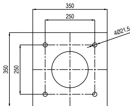
BASE TEMPLATE
